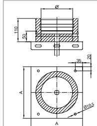
Tussenondersteuning met condensafvoer onder / ADWECO05
