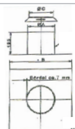
Platdakdoorvoer incl. stormkraag / ADWECO52H
