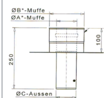
Verloop FLEX/TWIN / ATWIN466
