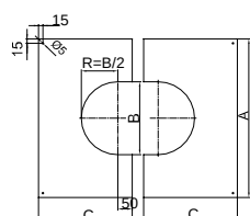
Centreerplaten (0° - 30°) 2-delig / ADWECO99V
